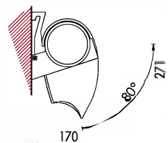
Pose de face 80° Montaje a pared 80°
